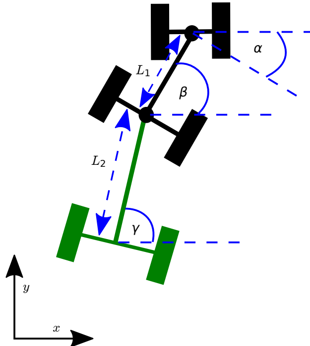
Abbildung 1: Skizze des Traktors mit Anhänger
