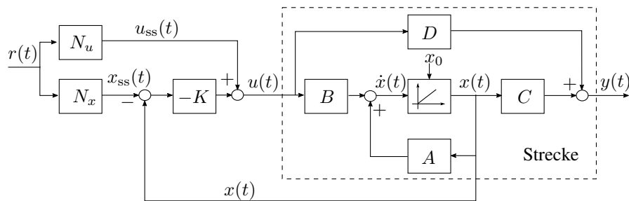
Abbildung 12.5: Linearer Zustandsregler mit Arbeitspunktwechsel.
