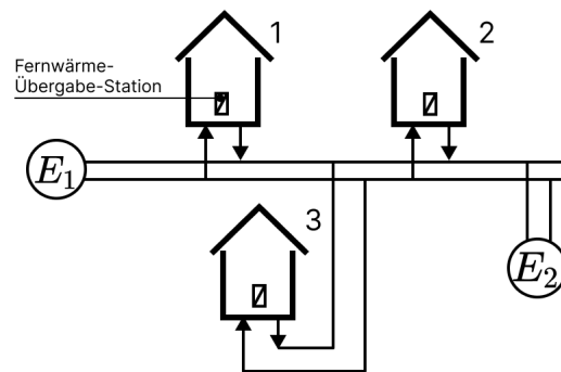
Abbildung A.11: Wärmeverbundnetz
