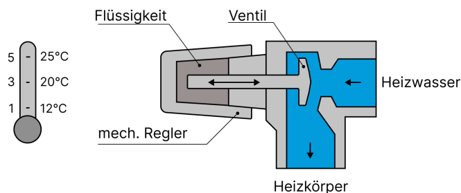
Abbildung A.1: Thermostat und Sollwertvorgabe
