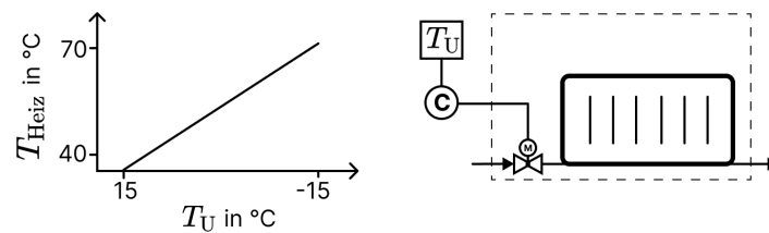
Abbildung A.4: Steuerung der Raumtemperatur mit Heizkurve
