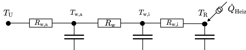
Abbildung A.7: Thermisches RC-Netzwerk des Gebäudemodells dritter Ordnung (3R3C)
