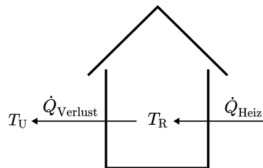
Abbildung A.5: Schema des Gebäudemodells erster Ordnung
