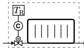
Abbildung A.3: Regelung der Raumtemperatur mit Software-Regler
