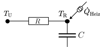
Abbildung A.6: Thermisches RC-Netzwerk erster Ordnung (1R1C) des Gebäudemodells
