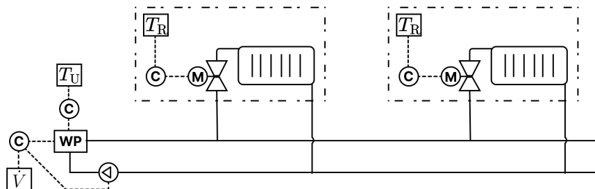
Abbildung A.10: Regelung mit einem Thermostatventil pro Raum und witterungsgeführter Vorlauftemperatur der Wärmepumpe
