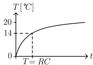
Abbildung A.9: Sprungantwort für Aufheizvorgang Beispielgebäude
