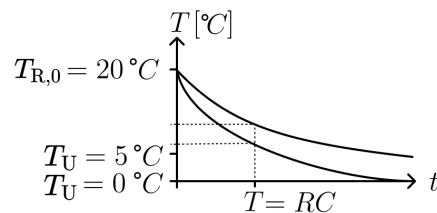
Abbildung A.8: Zeitliches Verhalten der Gebäudeabkühlung bei Heizungsausfall für T_U = 0\text{ °C} und T_U = 5\text{ °C}
